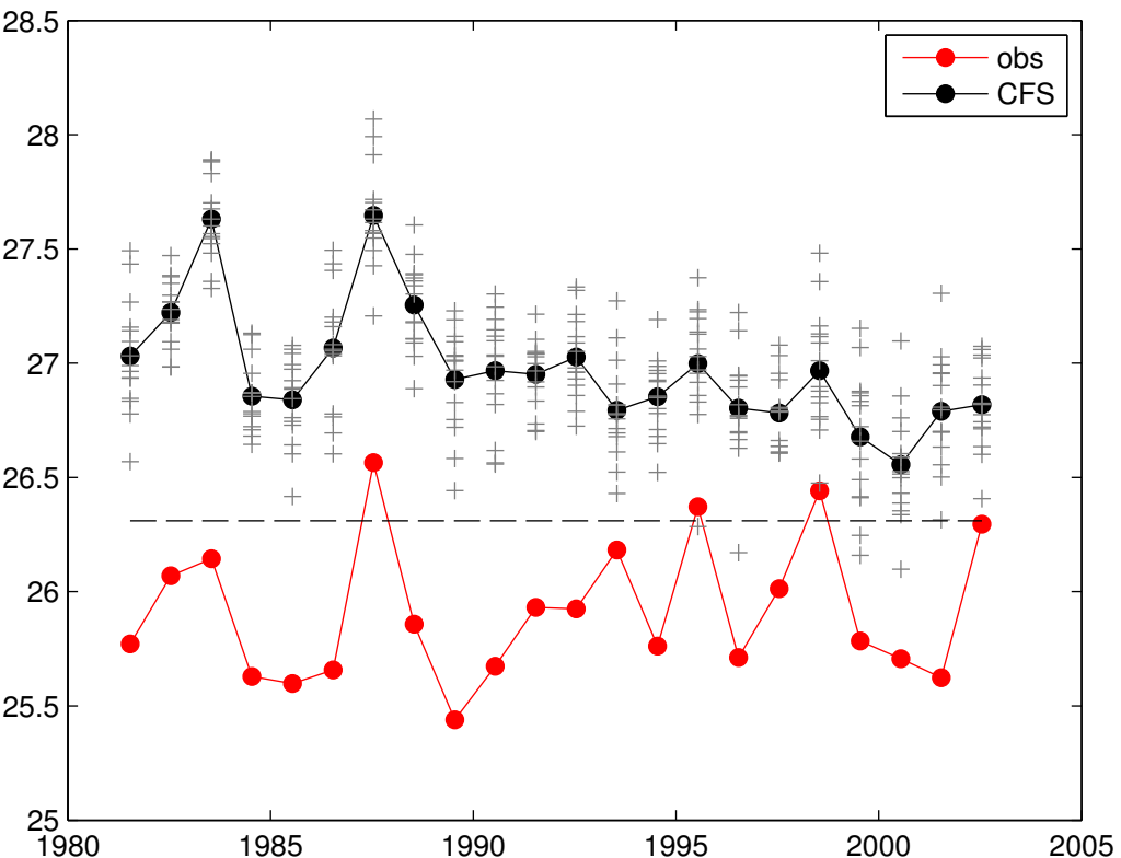
JJA t2m
