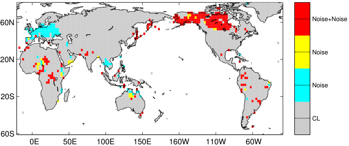
F-test
