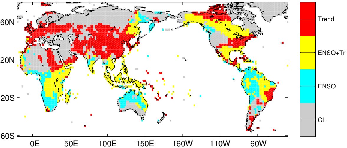
F-test
