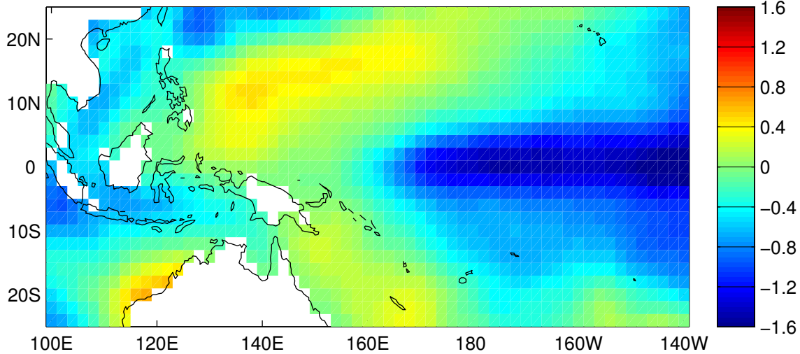
SST anomaly JFM 1971
