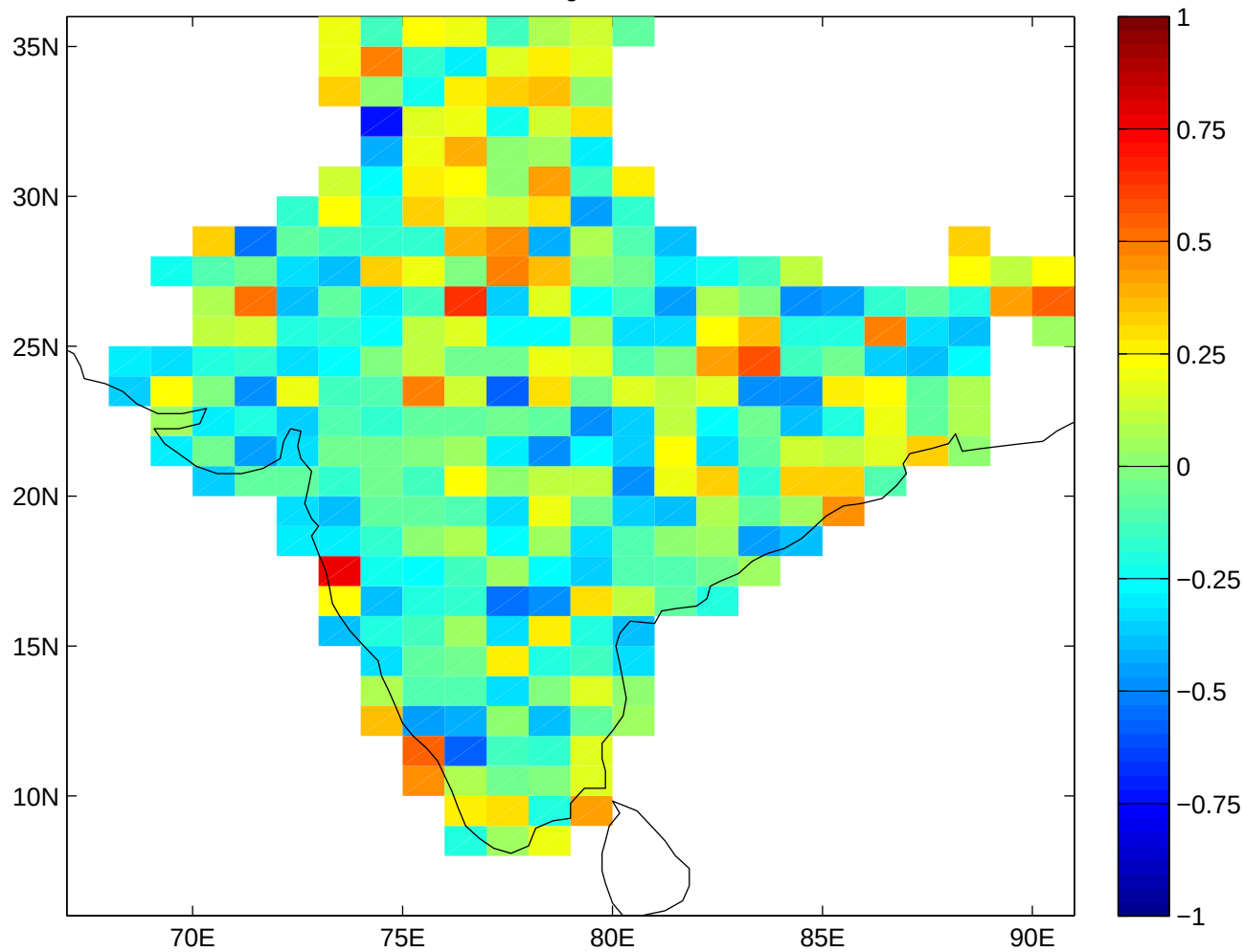
ECHAM4.5 GML g=-0.045 rms=8.1
