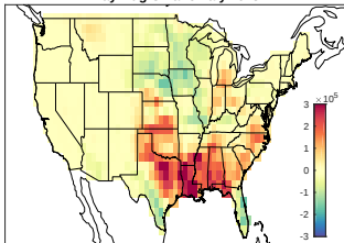
May-Aug CP anomaly 2013
