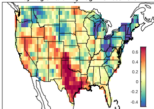
May-Aug CP and May-Aug PDO 2003-2016
