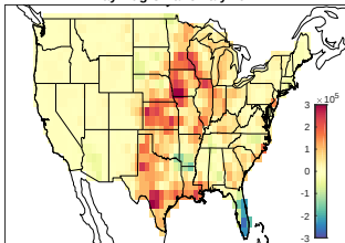
May-Aug CP anomaly 2011
