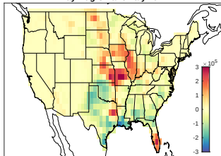
May-Aug CP anomaly 2014
