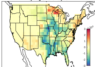
May-Aug CP anomaly 2012
