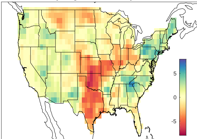
May-Aug PRCP anomaly 2008
