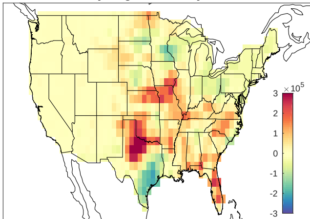
May-Aug CP anomaly 2006
