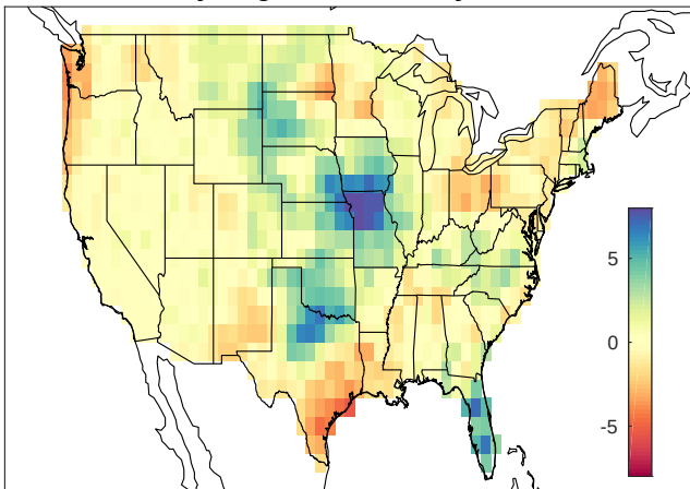
May-Aug PRCP anomaly 2006
