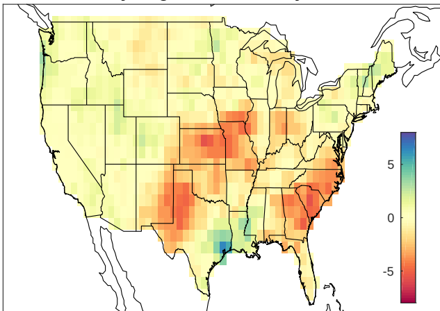
May-Aug cPRCP anomaly 2007
