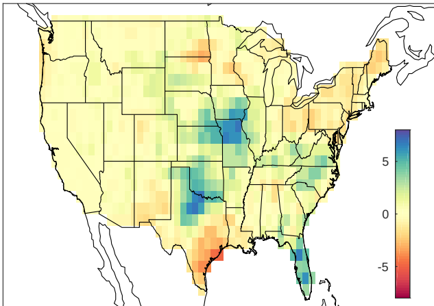
May-Aug cPRCP anomaly 2006
