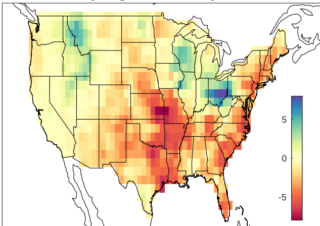
May-Aug PRCP anomaly 2004
