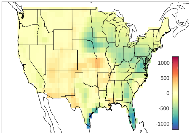
May-Aug CAPE anomaly 2005
