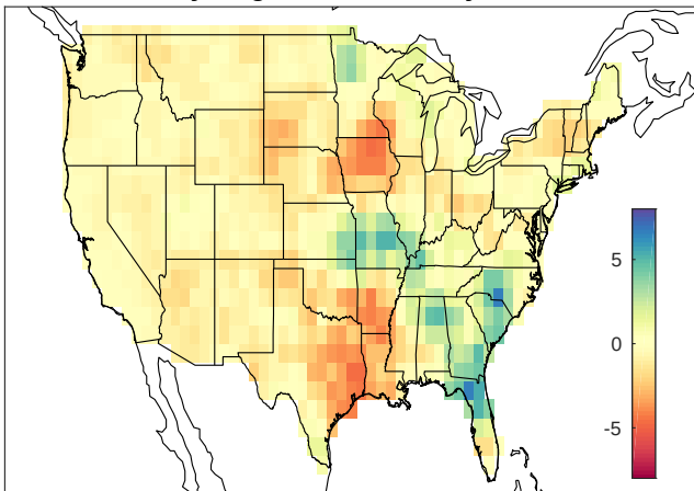
May-Aug cPRCP anomaly 2009
