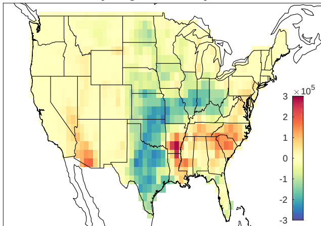
May-Aug CP anomaly 2008
