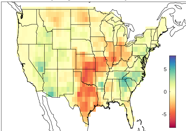
May-Aug cPRCP anomaly 2008
