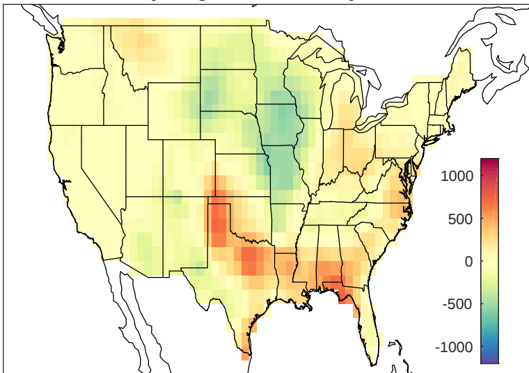
May-Aug CAPE anomaly 2013
