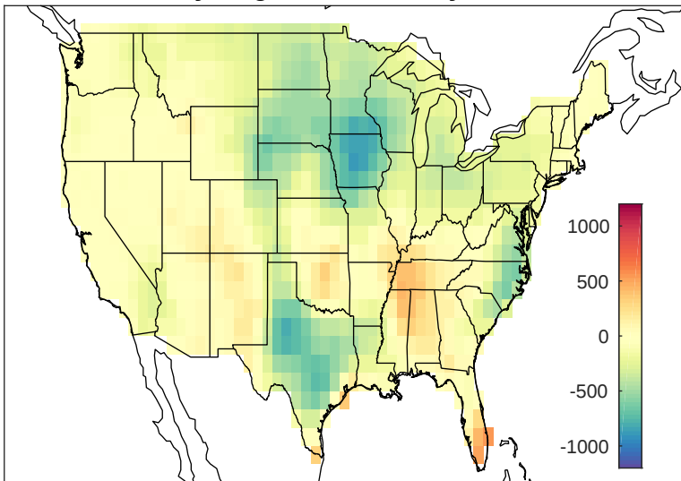
May-Aug CAPE anomaly 2009
