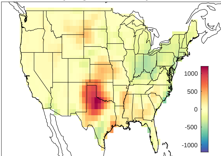
May-Aug CAPE anomaly 2006
