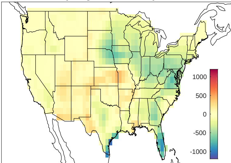
May-Aug CAPE anomaly 2005
