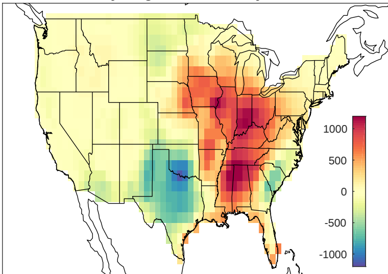
May-Aug CAPE anomaly 2004
