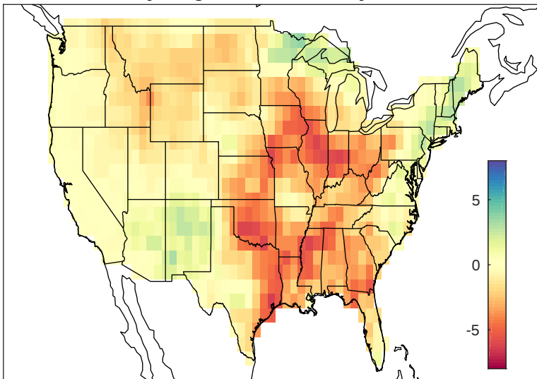
May-Aug cPRCP anomaly 2012
