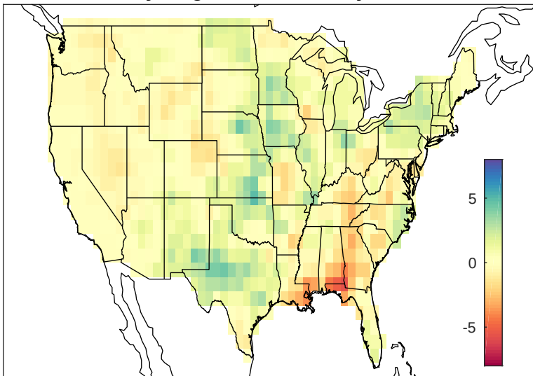
May-Aug cPRCP anomaly 2010
