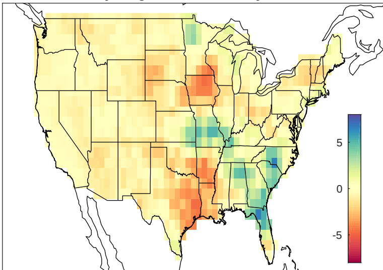
May-Aug cPRCP anomaly 2009
