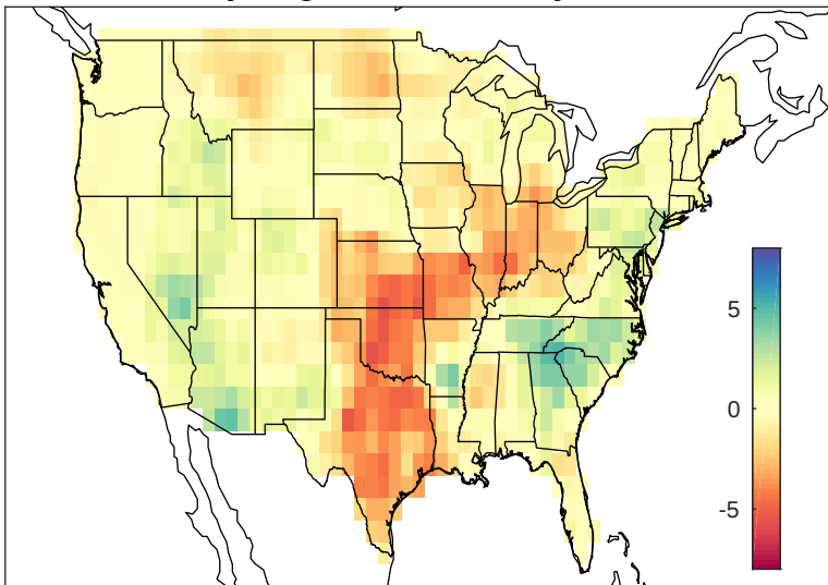
May-Aug cPRCP anomaly 2008
