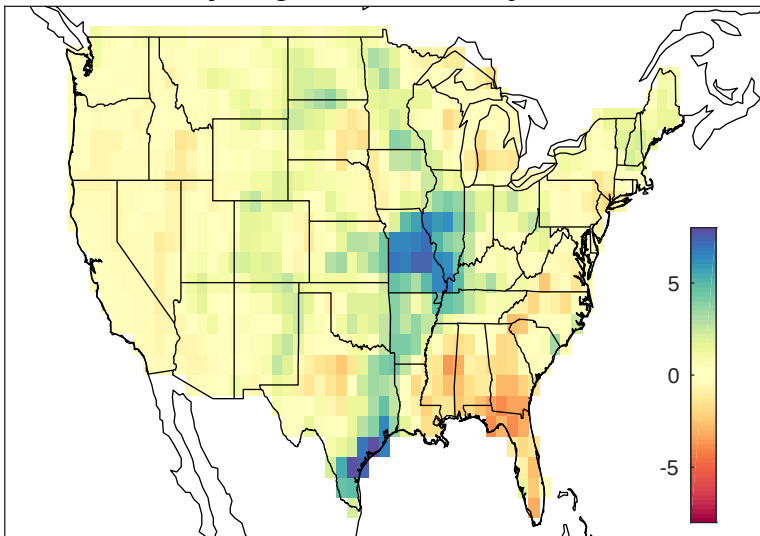
May-Aug cPRCP anomaly 2005
