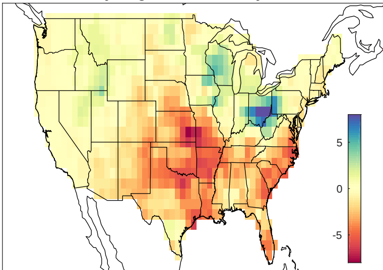
May-Aug cPRCP anomaly 2004
