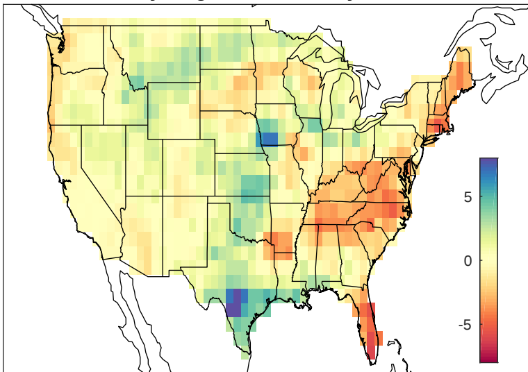
May-Aug PRCP anomaly 2011
