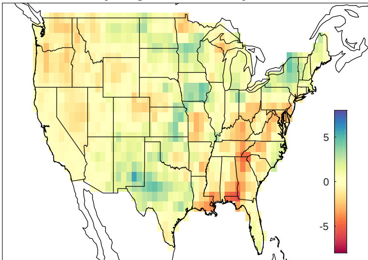
May-Aug PRCP anomaly 2010
