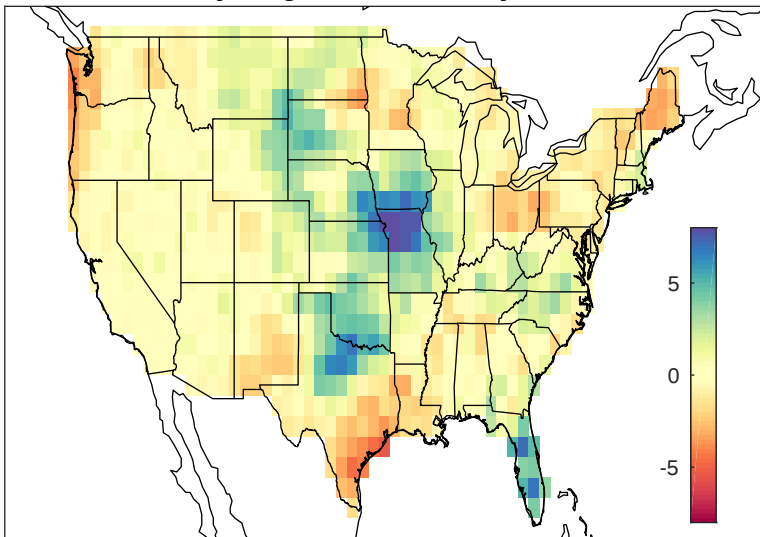
May-Aug PRCP anomaly 2006
