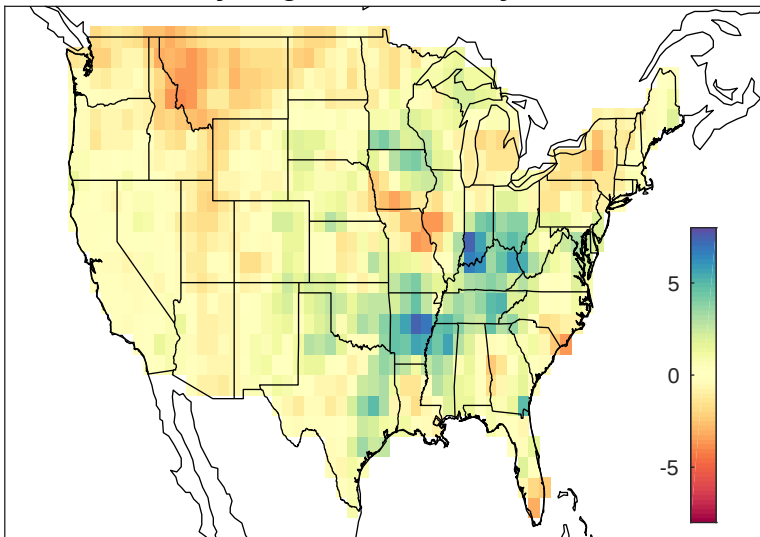
May-Aug PRCP anomaly 2003
