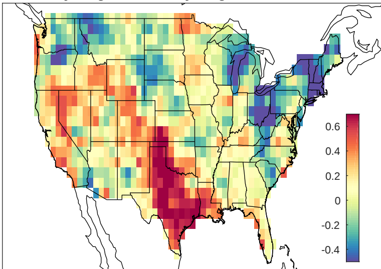
May-Aug CP and May-Aug PDO 2003-2016
