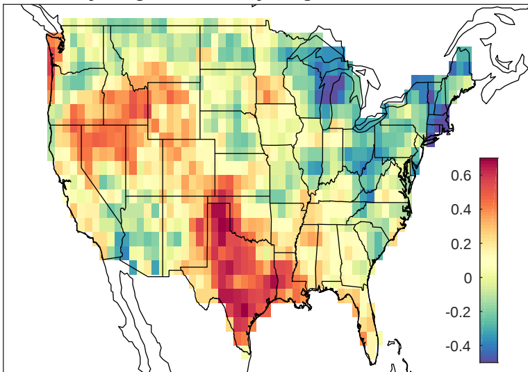
May-Aug CP and May-Aug PDO 1996-2016
